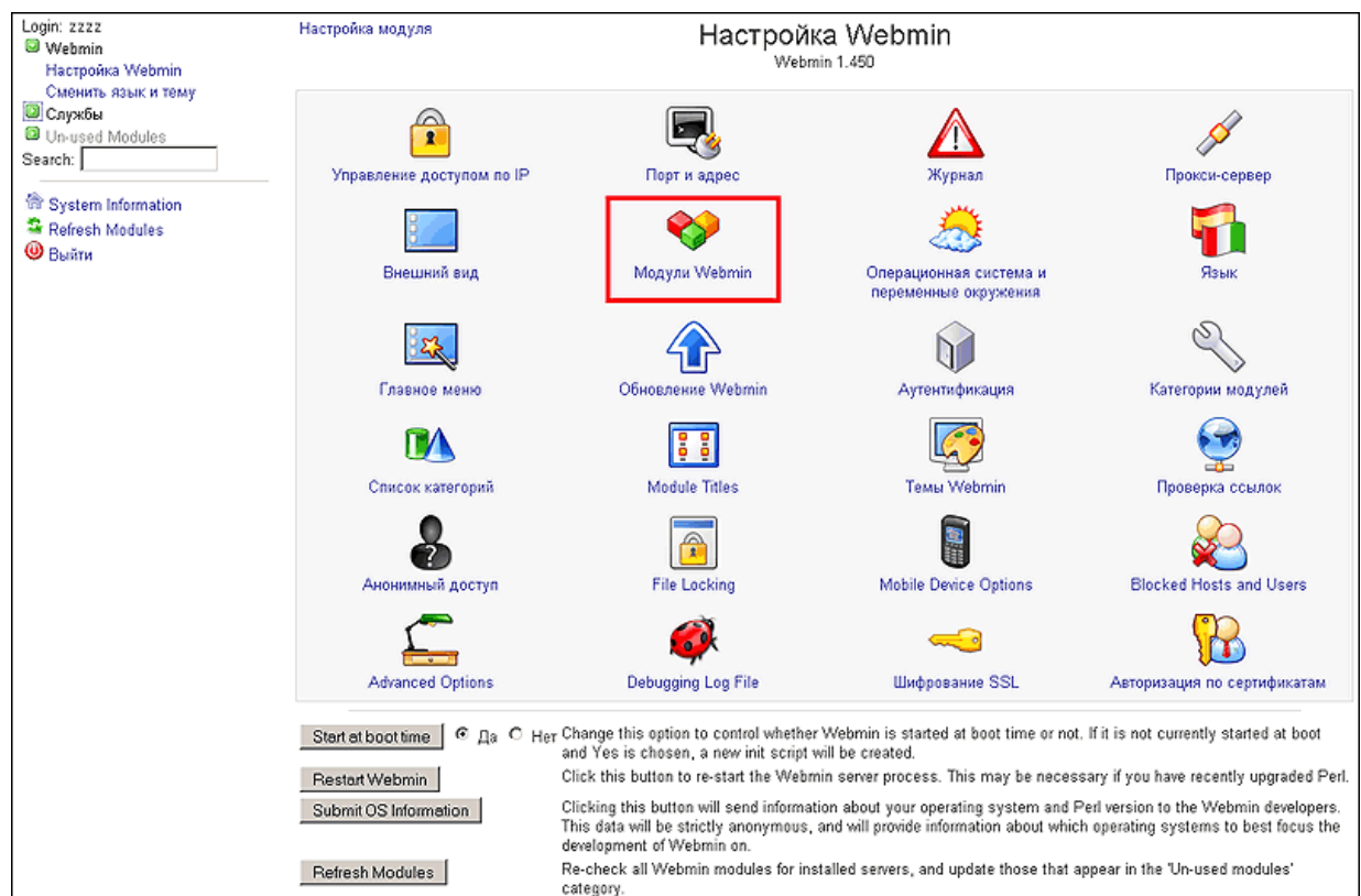
Рис. 19. Настройка Webmin
