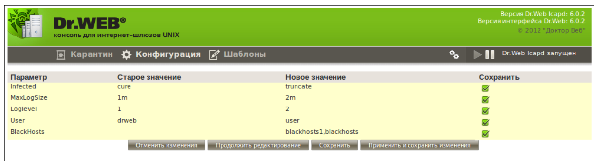
Рис. 24. Страница предпросмотра
