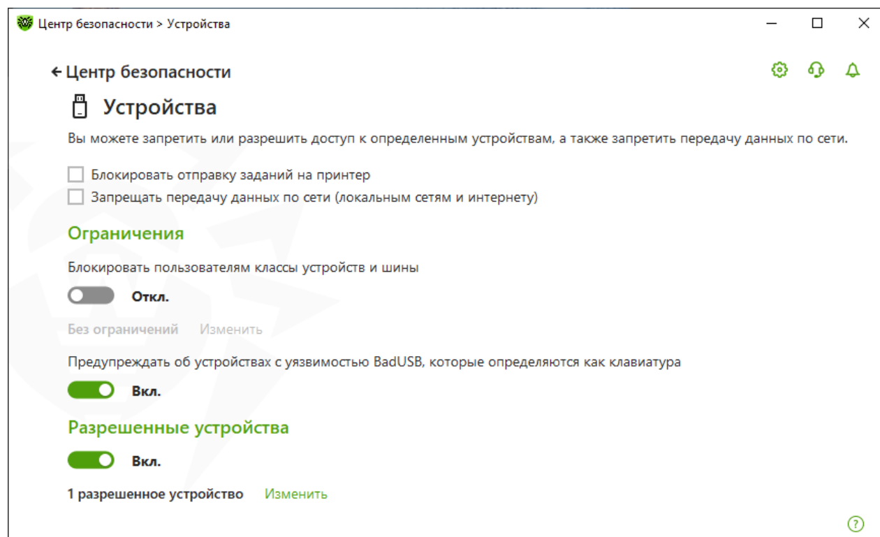
Рисунок 70. Параметры блокировки устройств
