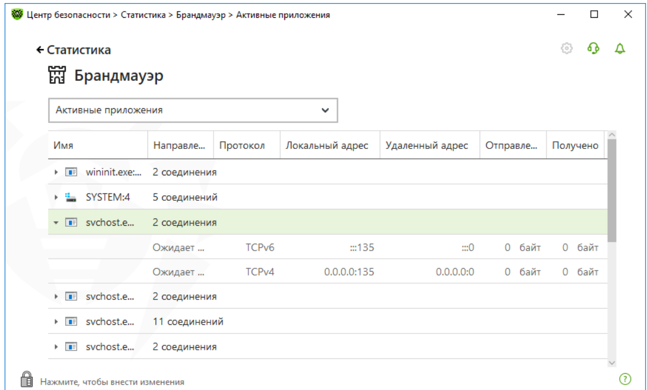
Рисунок 100. Окно статистики сетевой активности
