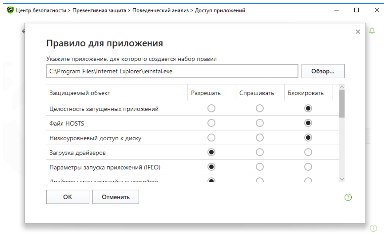
Рисунок 66. Добавление набора правил для приложения
