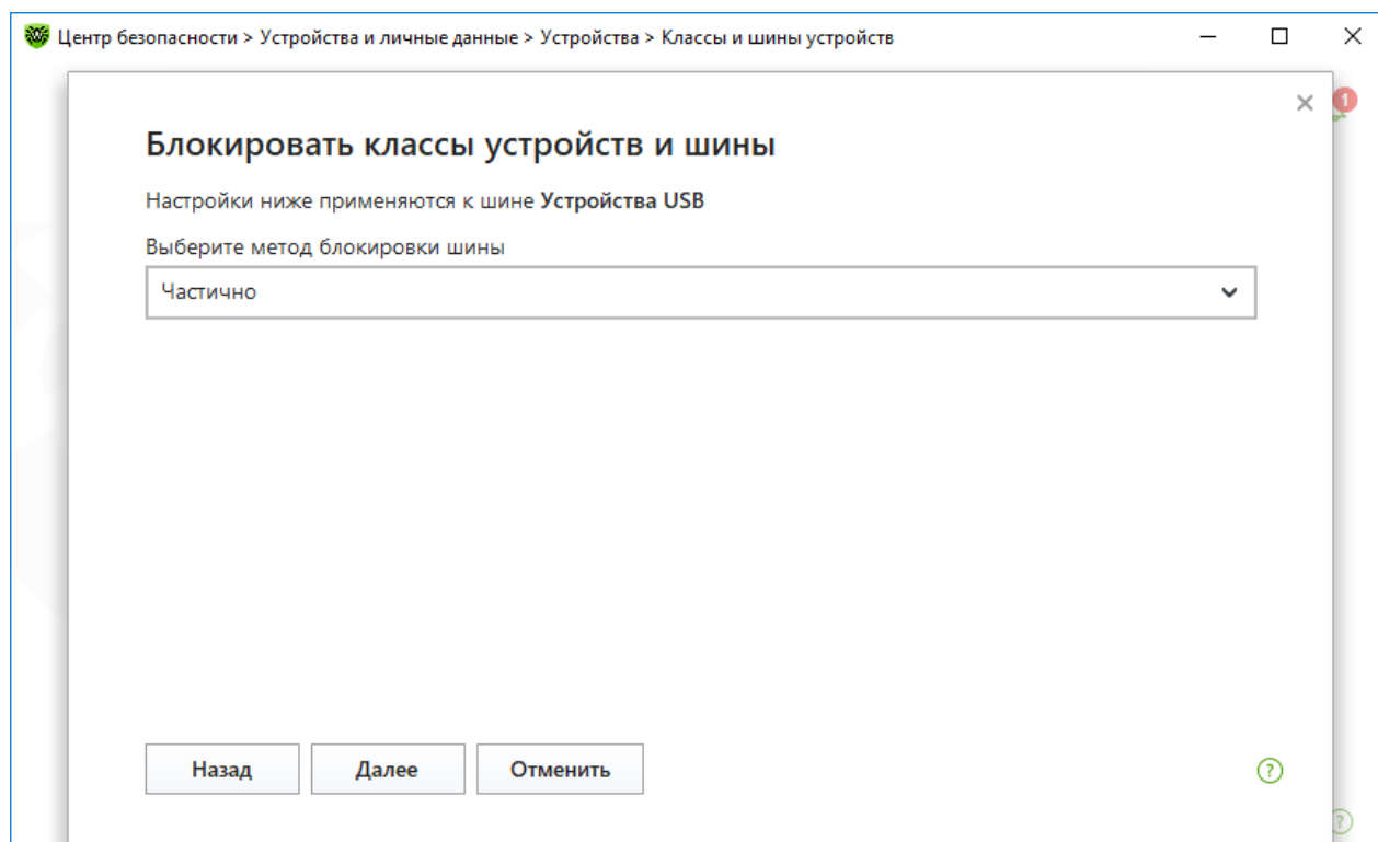
Рисунок 75. Выбор метода блокировки шины
