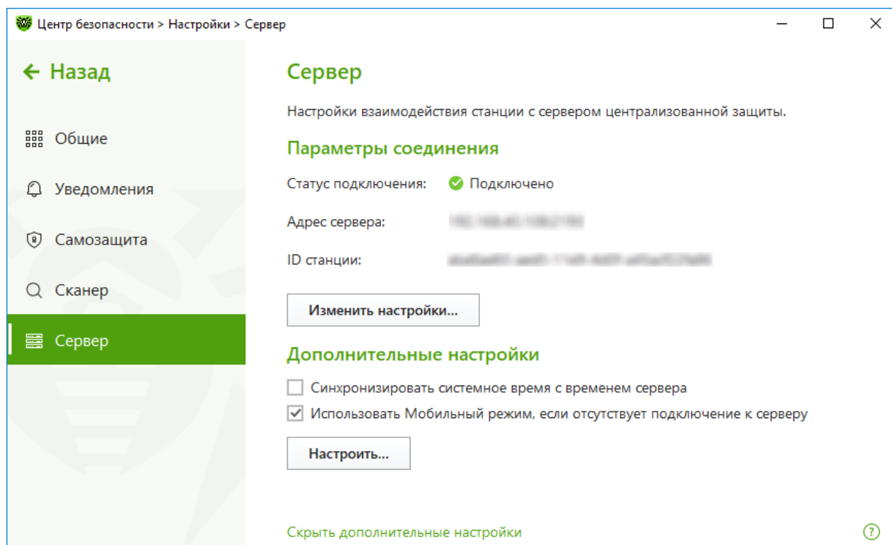
Рисунок 26. Настройки соединения станции
