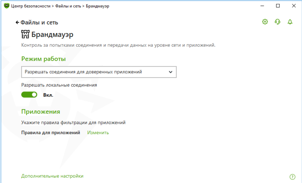
Рисунок 43. Параметры Брандмауэра
