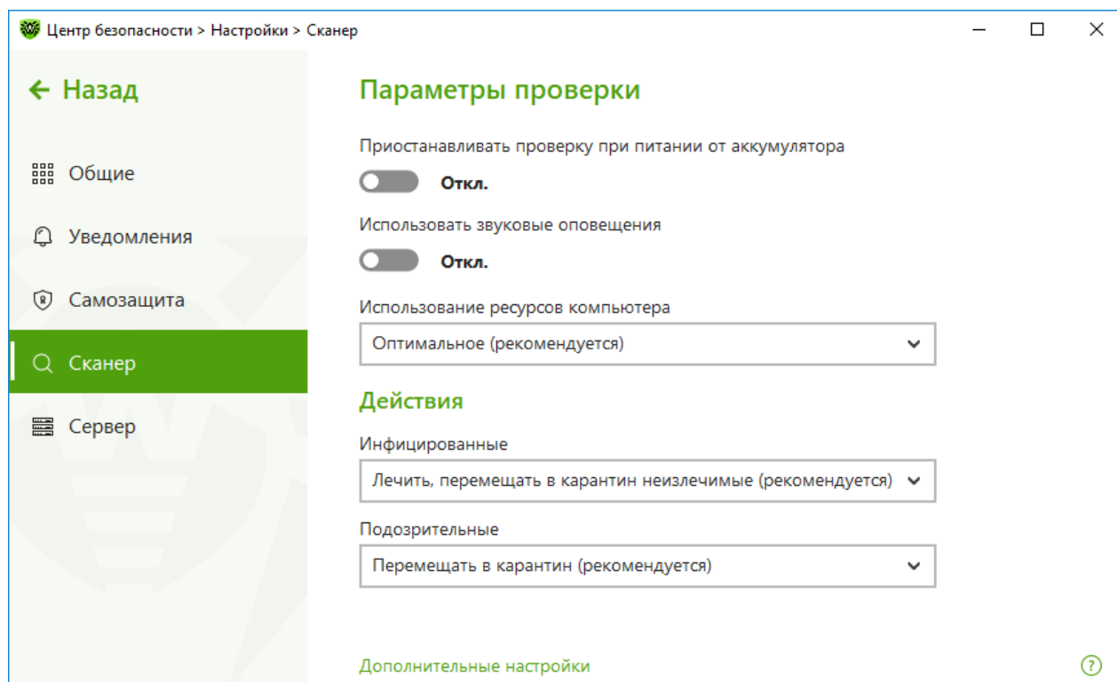
Рисунок 25. Настройка Сканера
