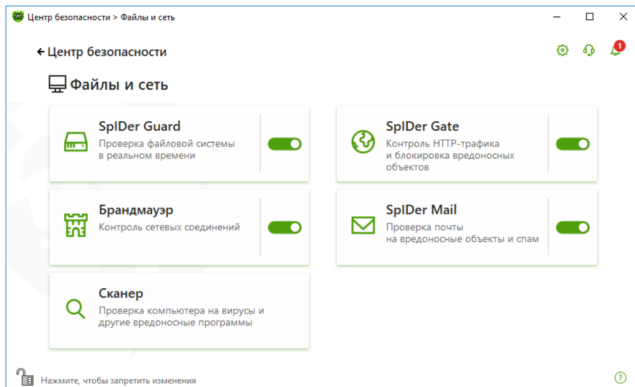
Рисунок 42. Включение/отключение Брандмауэра
