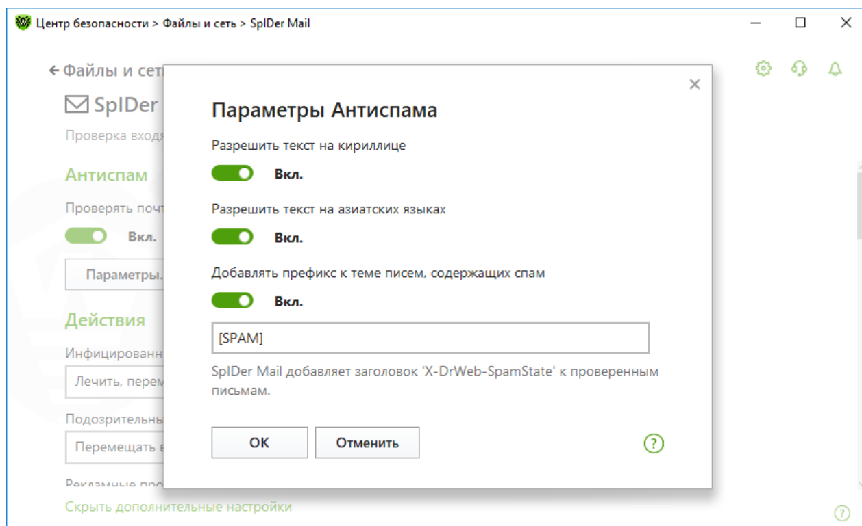
Рисунок 41. Параметры Антиспама
