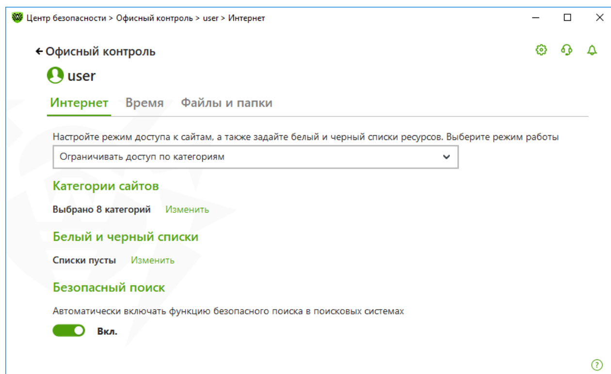
Рисунок 83. Параметры Офисного контроля
