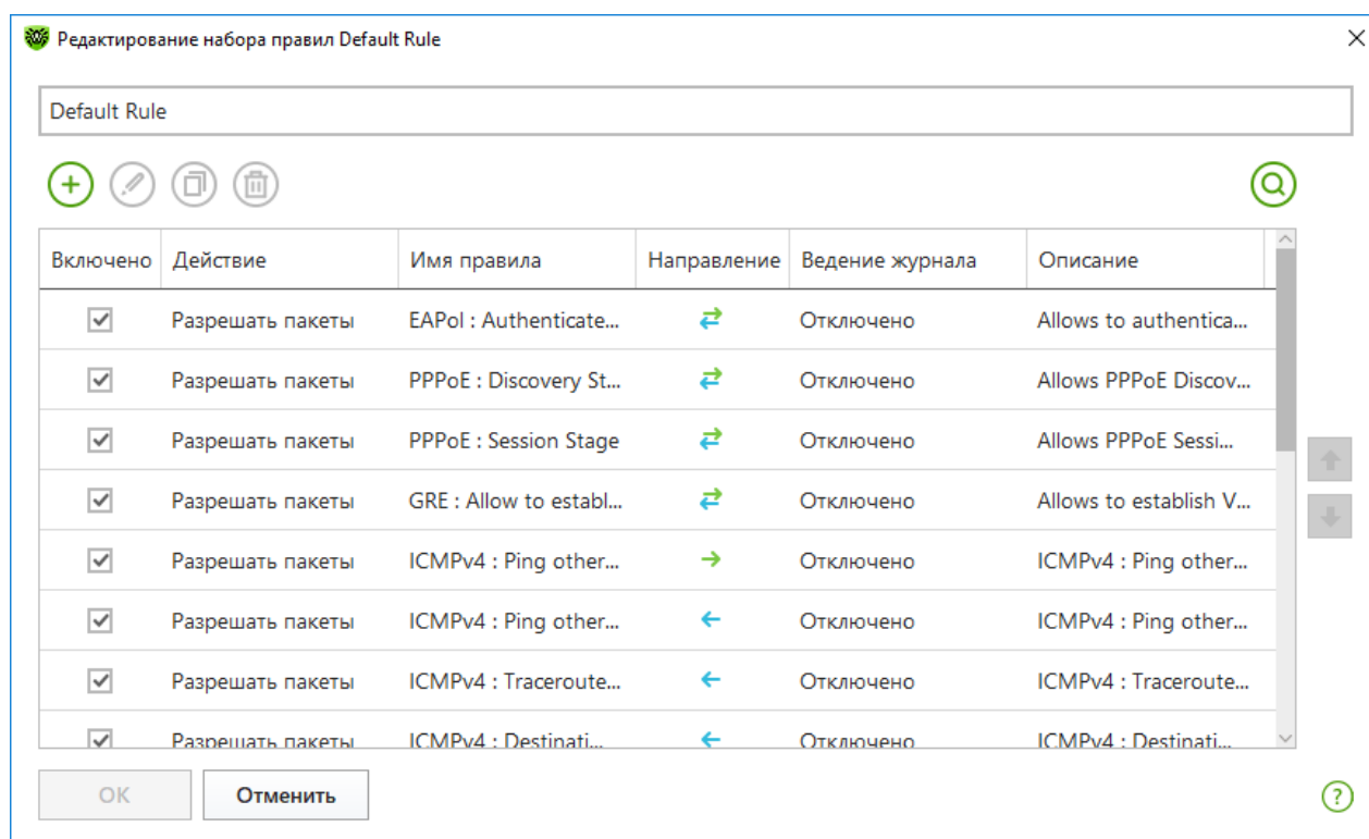
Рисунок 49. Набор правил фильтрации пакетов
