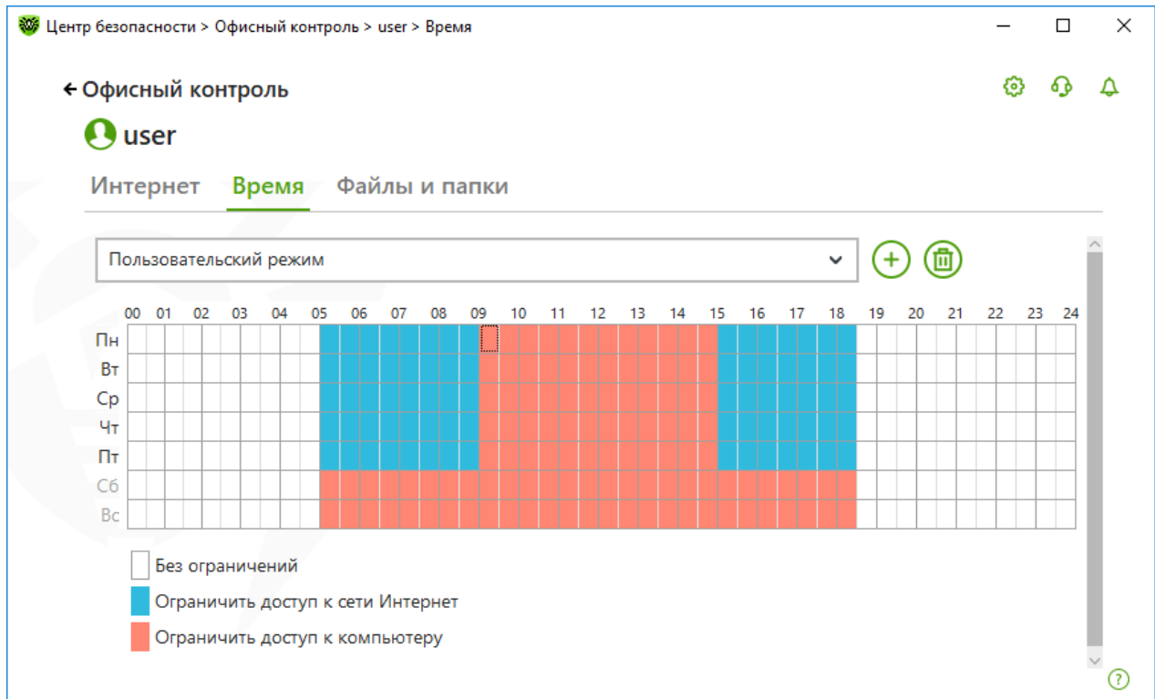
Рисунок 87. Таблица времени работы за компьютером и в интернете
