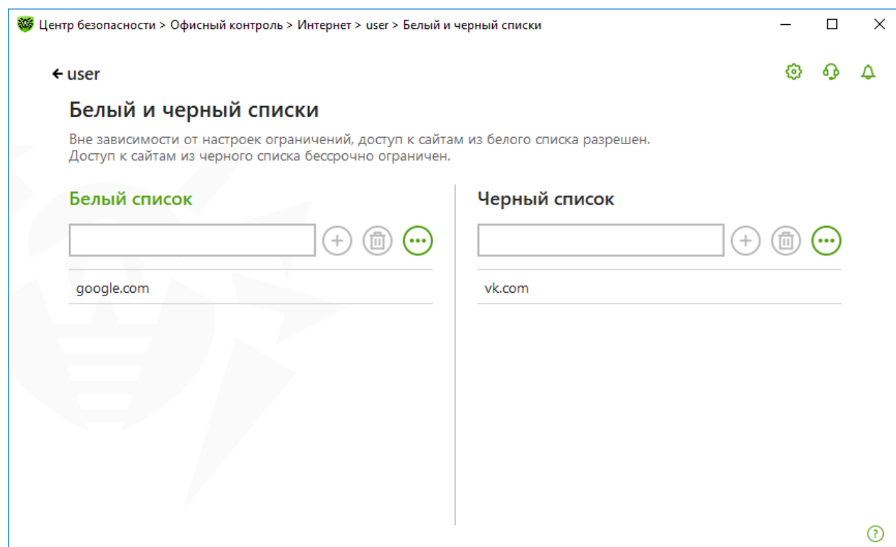
Рисунок 86. Настройка белого и черного списков Офисного контроля
