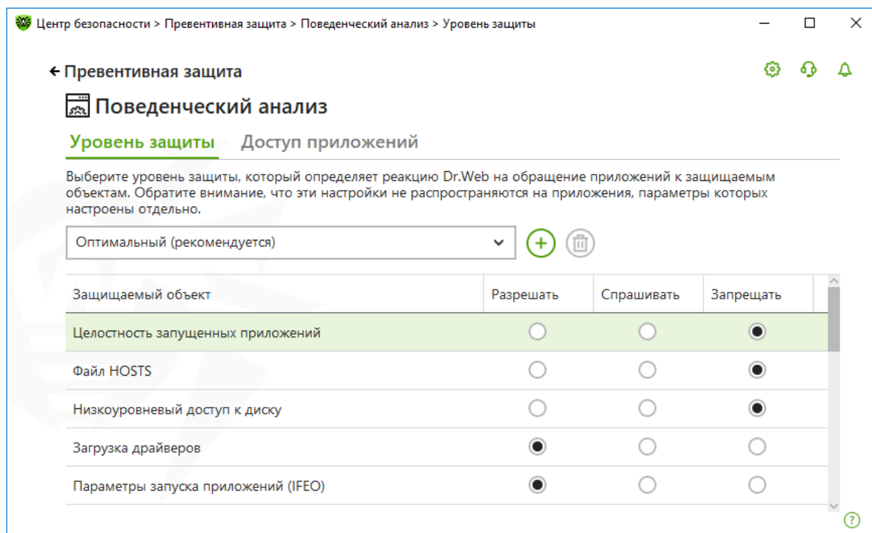
Рисунок 62. Параметры Поведенческого анализа
