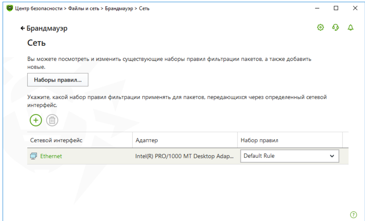
Рисунок 47. Наборы правил для сетевых интерфейсов
