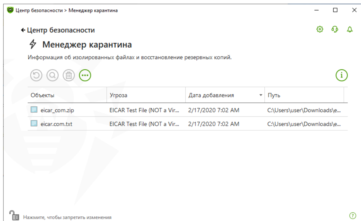
Рисунок 89. Объекты в карантине
