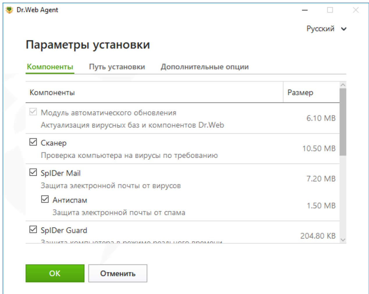
Рисунок 9. Параметры установки
