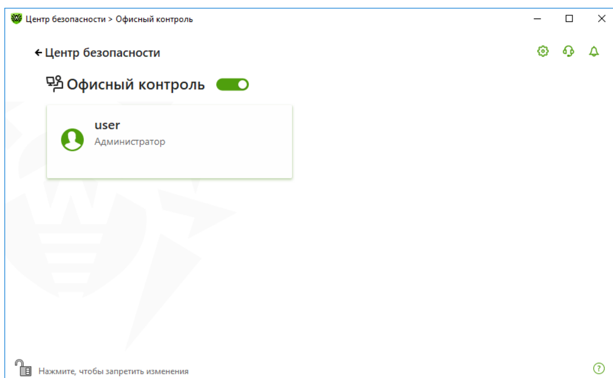
Рисунок 82. Офисный контроль
