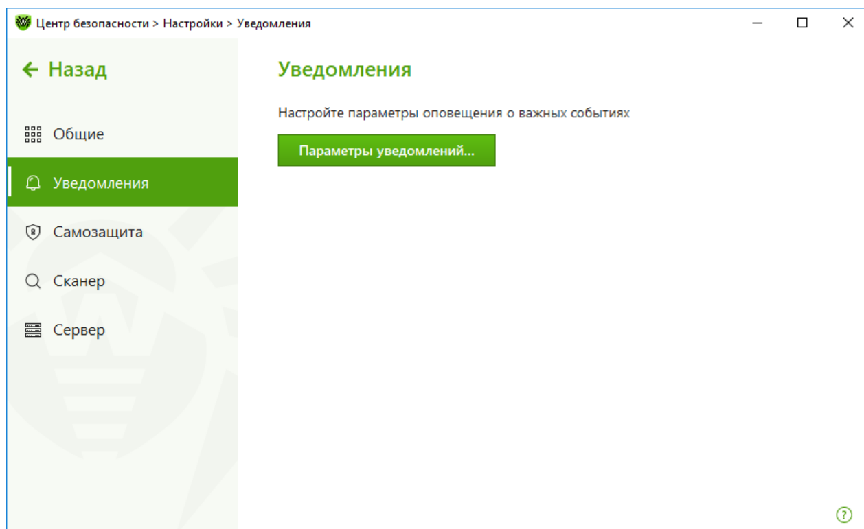
Рисунок 23. Настройки уведомлений
