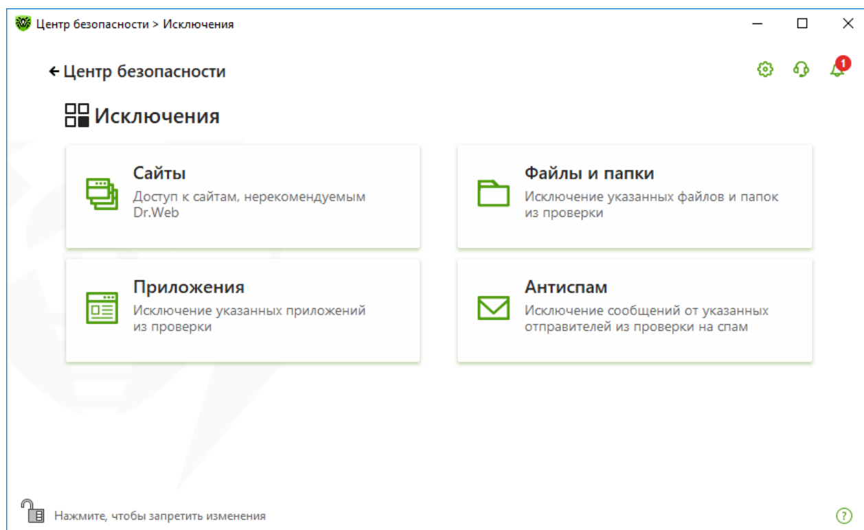
Рисунок 90. Окно Исключения
