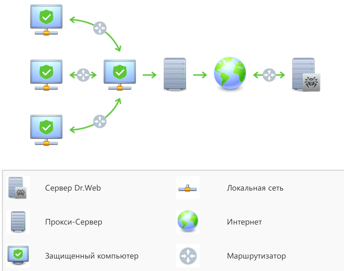
Рисунок 11-1. Схема антивирусной сети при использовании Прокси-сервера
